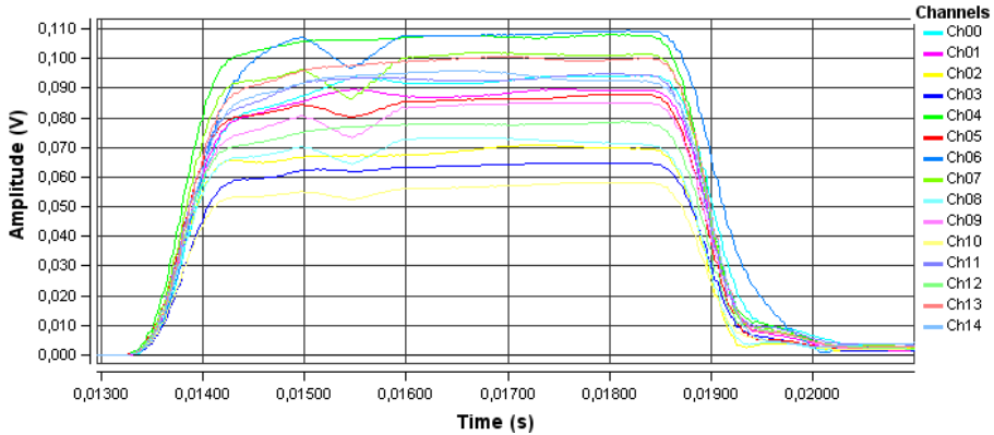
Fig. 3.2. Tx module values
