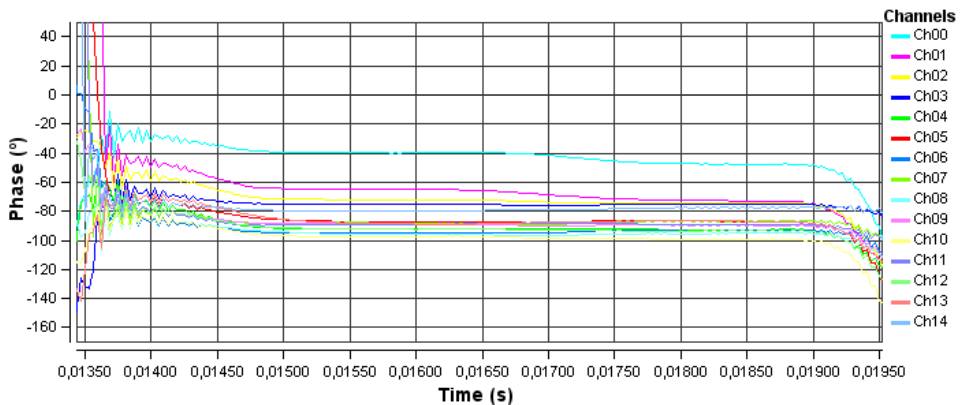
Fig. 4.2. Rx phase values
