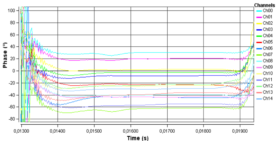
Fig. 3.3. Tx phase values
